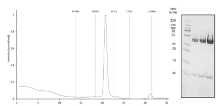
G-protein: Gαq-β-γ
